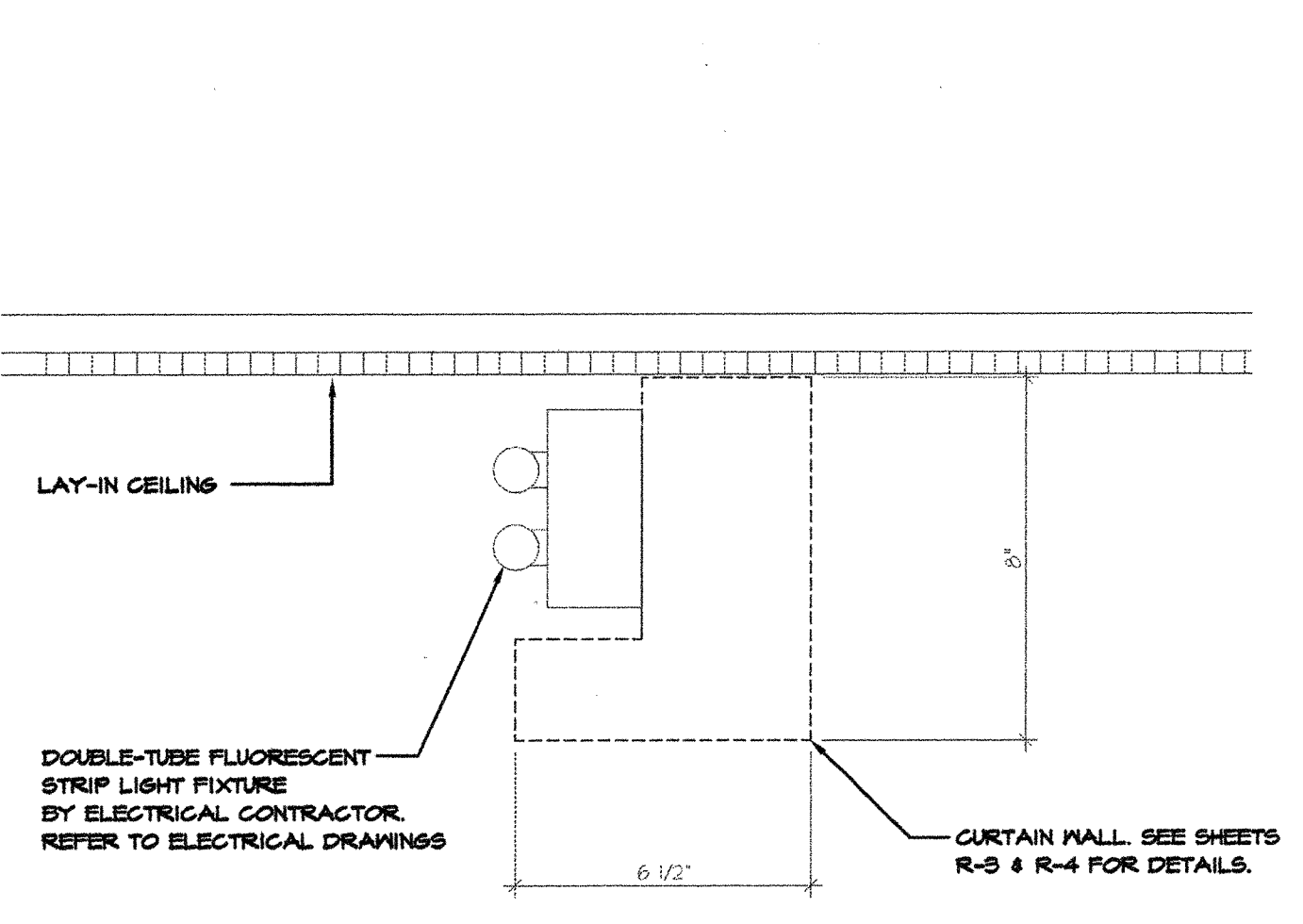
E LIGHTING SECTION SCALE: 1/2" = 1'-0"
