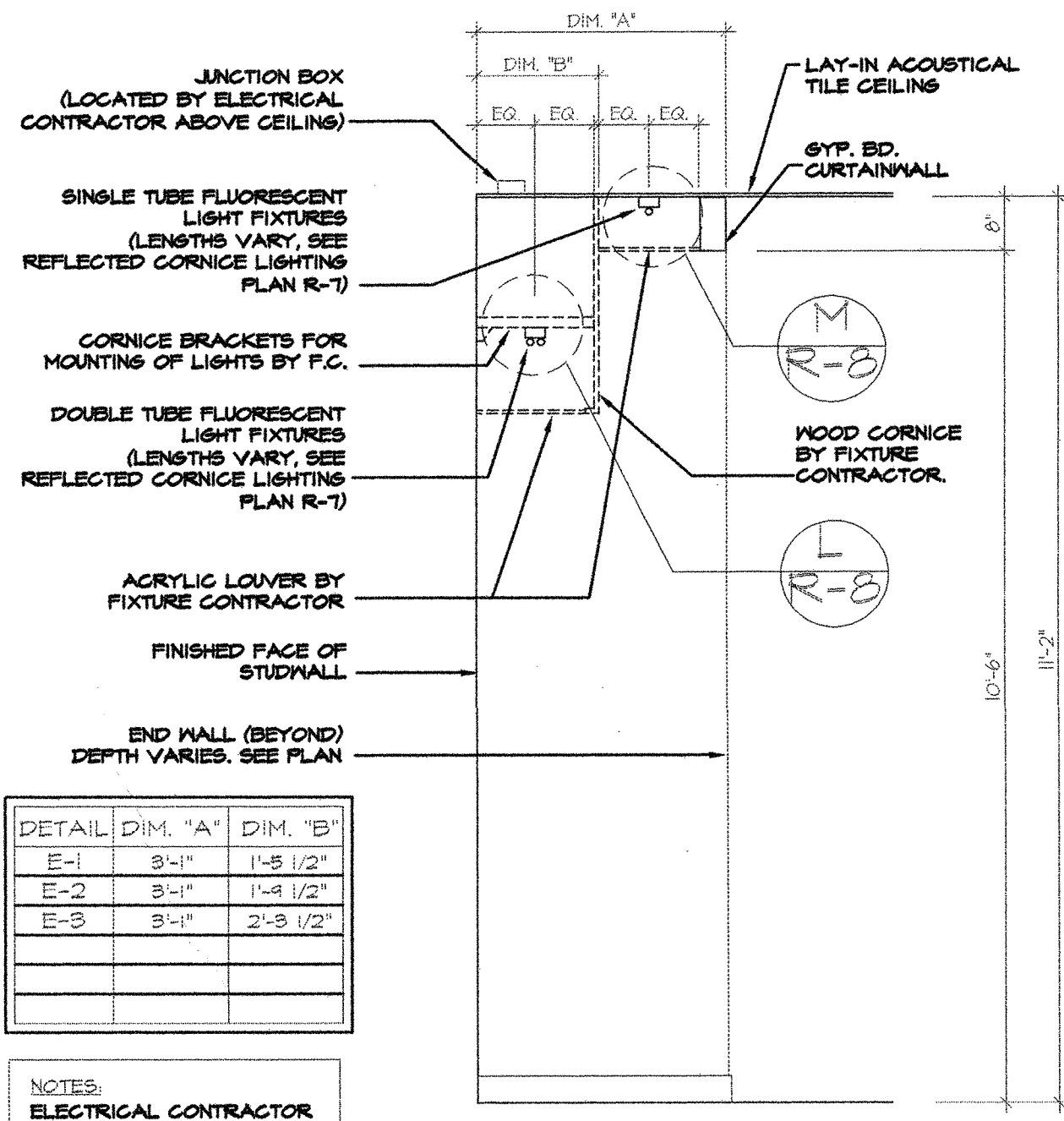
E LIGHTING SECTION SCALE: 1/2" = 1'-0"
