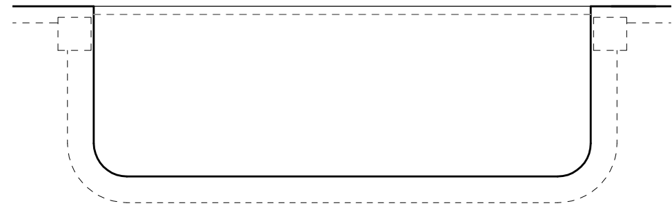
POOL SPA SECTION 3 SCALE: 1/4" = 1'-0"
