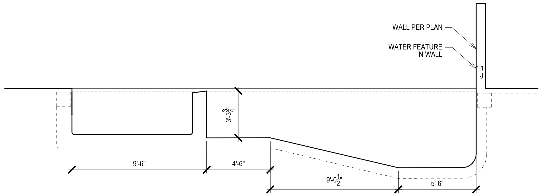
POOL SPA SECTION 2 SCALE: 1/4" = 1'-0"
