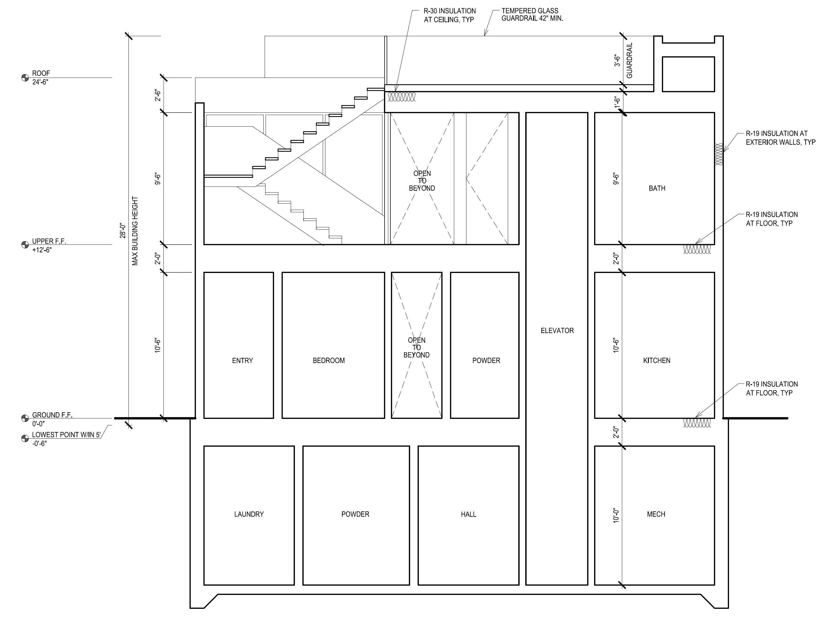
N-S SECTION 2 SCALE: 1/4"-1'-0"
