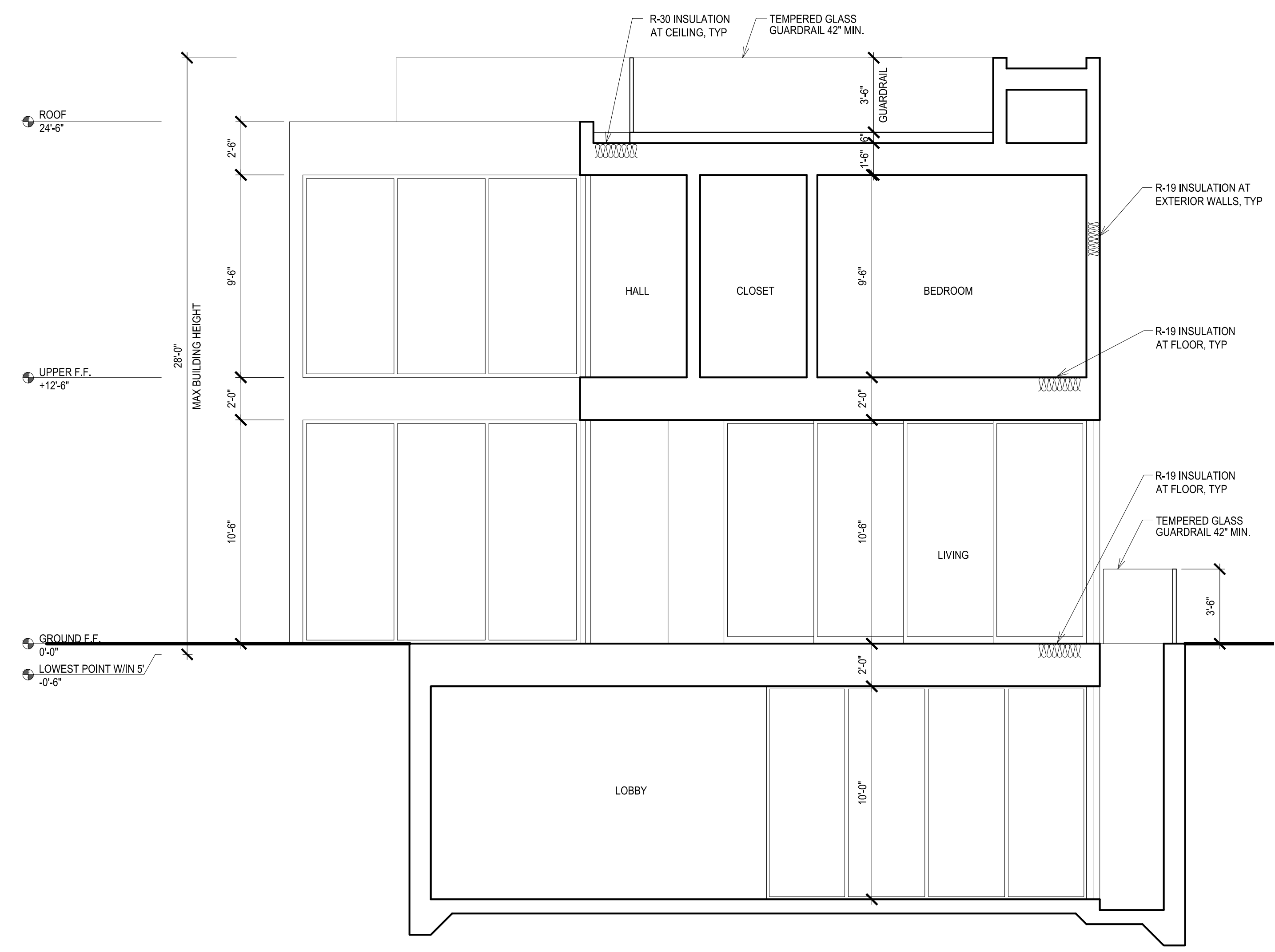
N-S SECTION 3 SCALE: 1/4"-1'-0"
