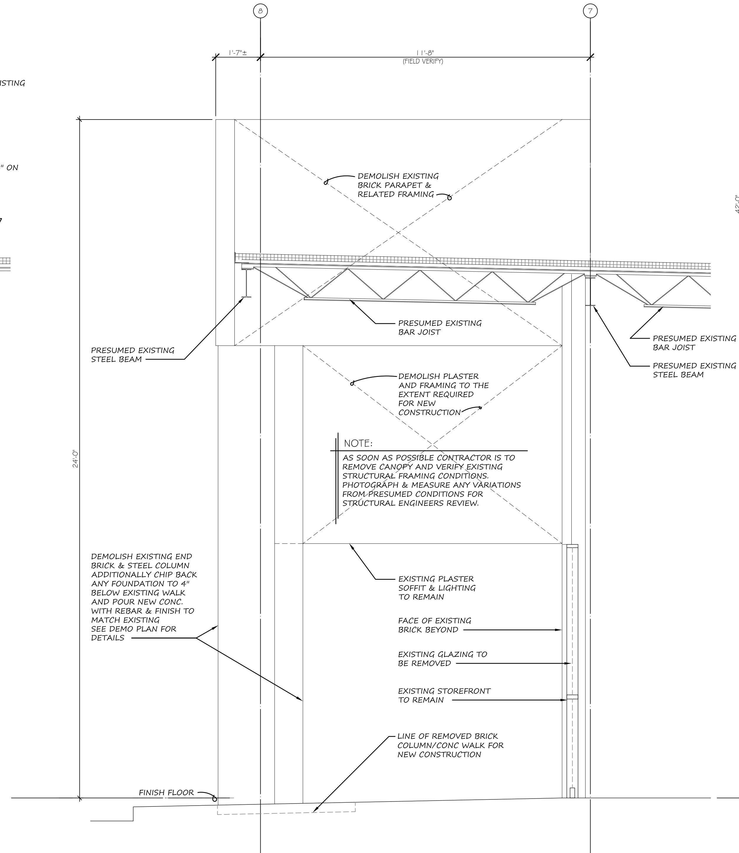
2 | EXISTING CANOPY SECTION A4-1 | SCALE: 1/2" = 1'-0"
