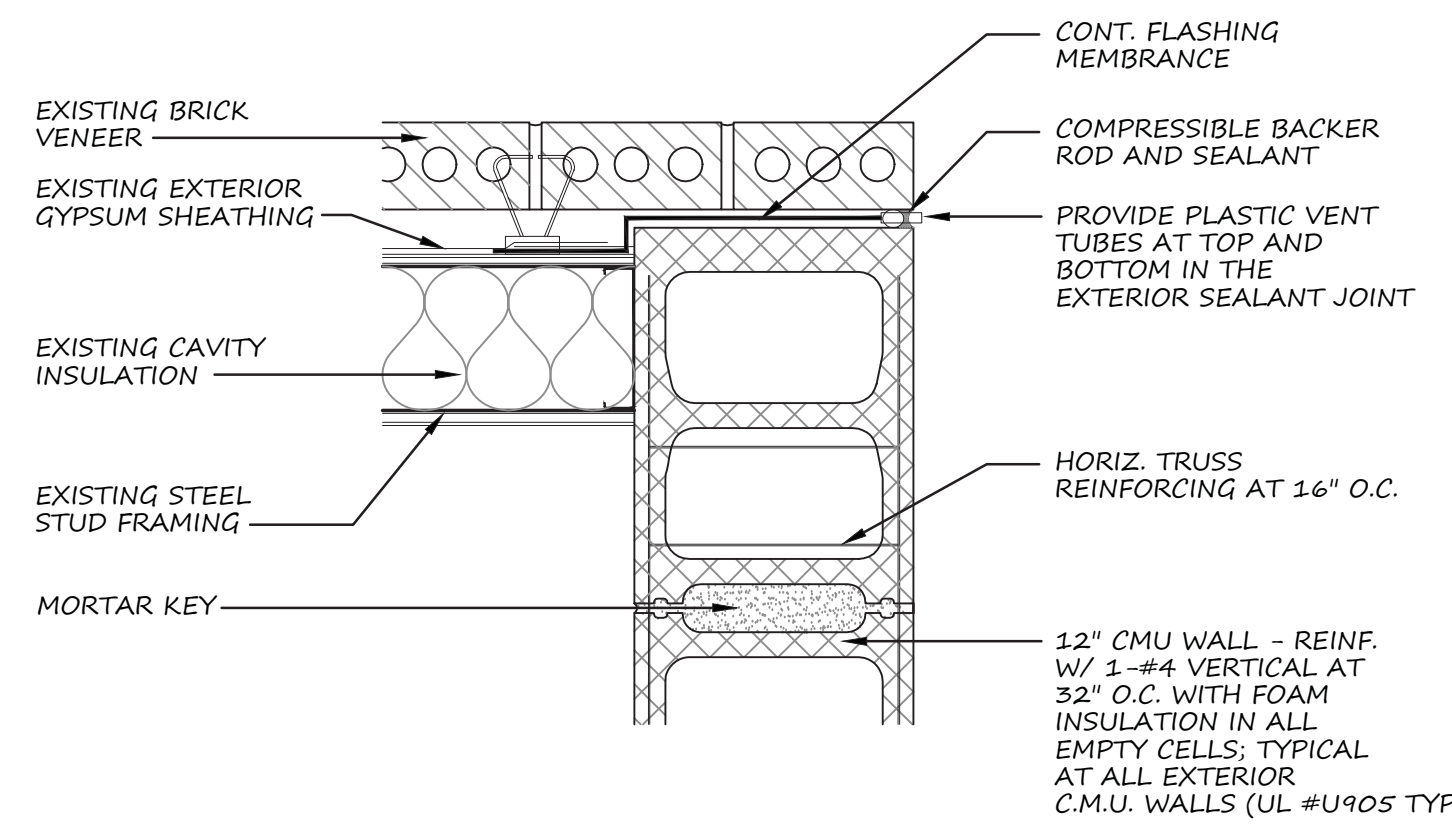
2 PLAN DETAIL A4-8 SCALE: 1 1/2" = 1'-0"
