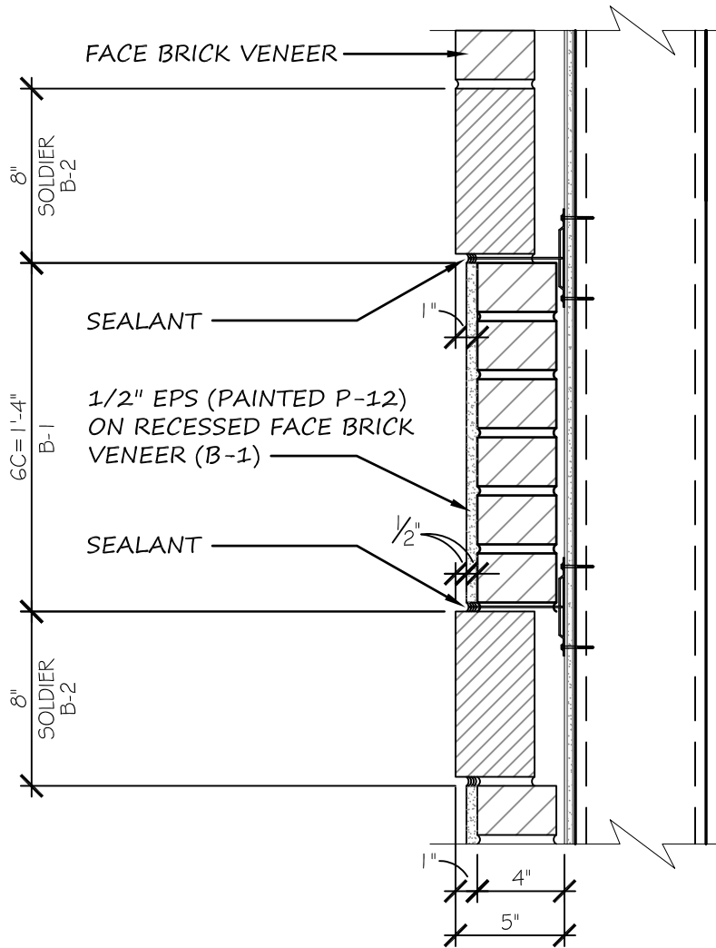
1 | BASE DETAIL A-SK-05 | SCALE: 1 1/2" = 1'-0"
