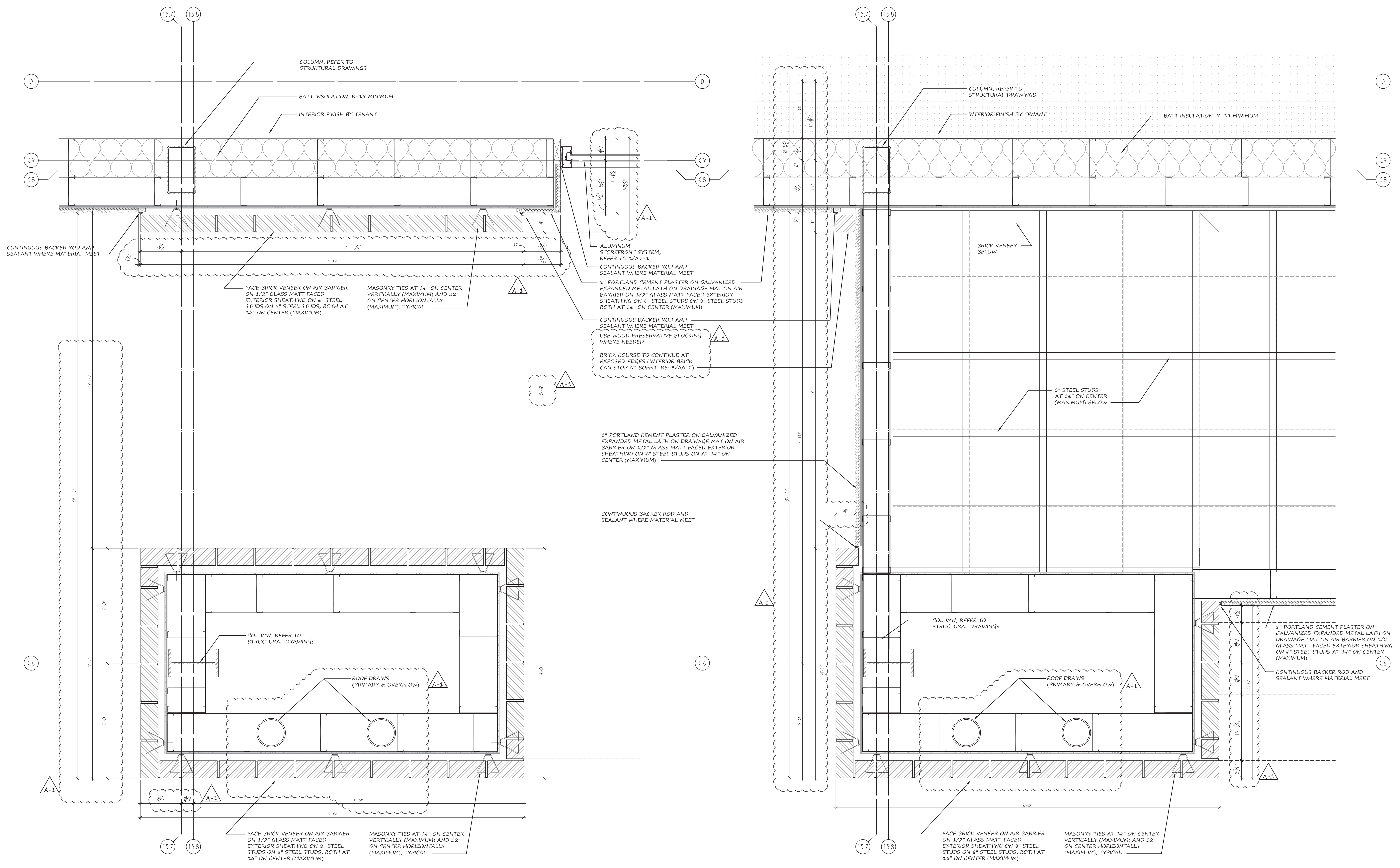
1 PLAN DETAIL A5-2 SCALE: 1 1/2" = 1'-0"
