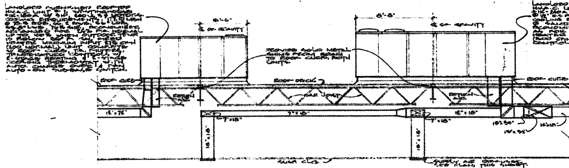
SECTION SCALE: 1/4" = 1'-0"
